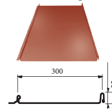
Click SRP 300
